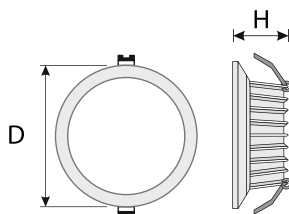
Рис.1. Габаритные размеры
